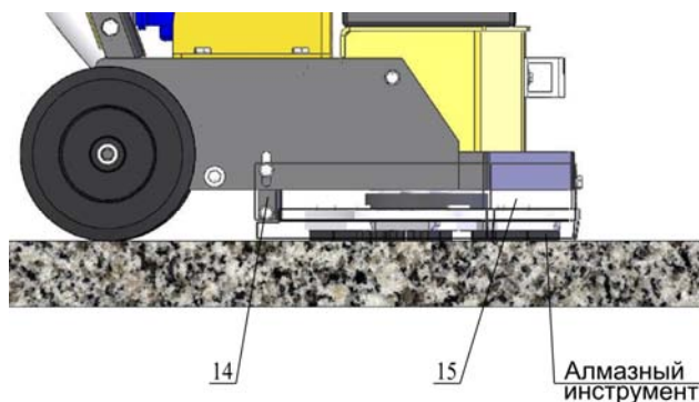
Новый комплект алмазного инструмента
