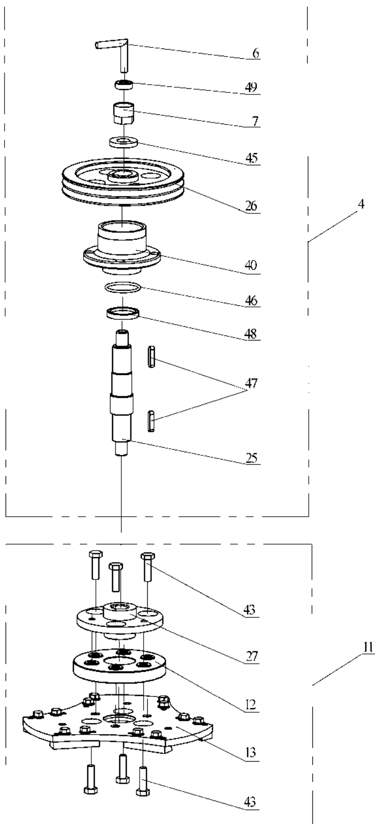
Рисунок 14 – Шпиндель и траверса шлифовальная
